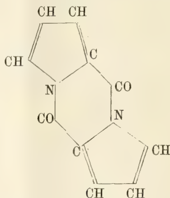
pirocolla ordinaria (imminidride dell'acido \alpha -carbopirrolico).
